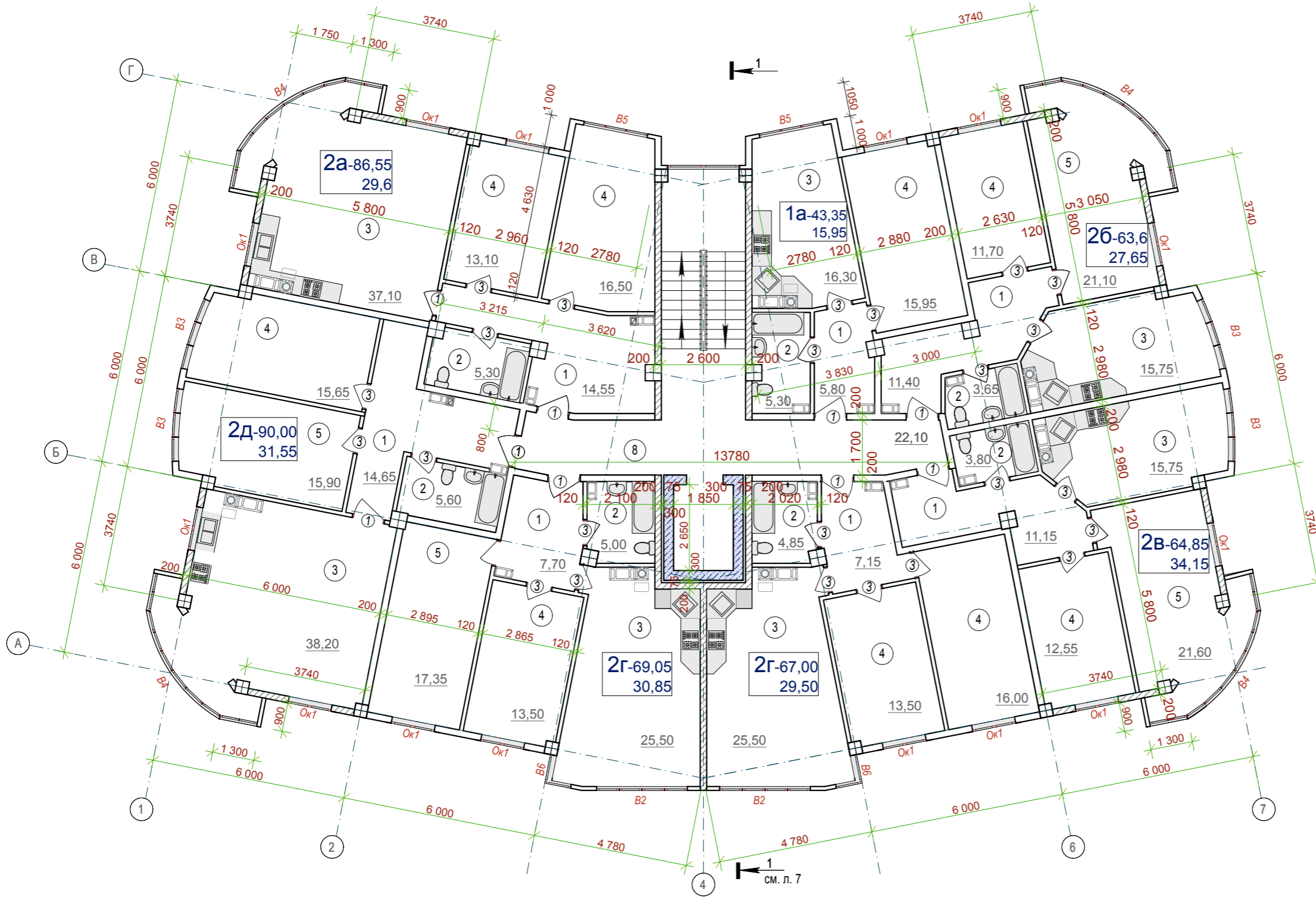
План на отм. 6.600-19.800
